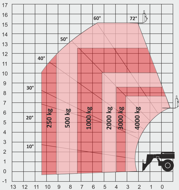
Диаграмма грузоподъемности на колесах
