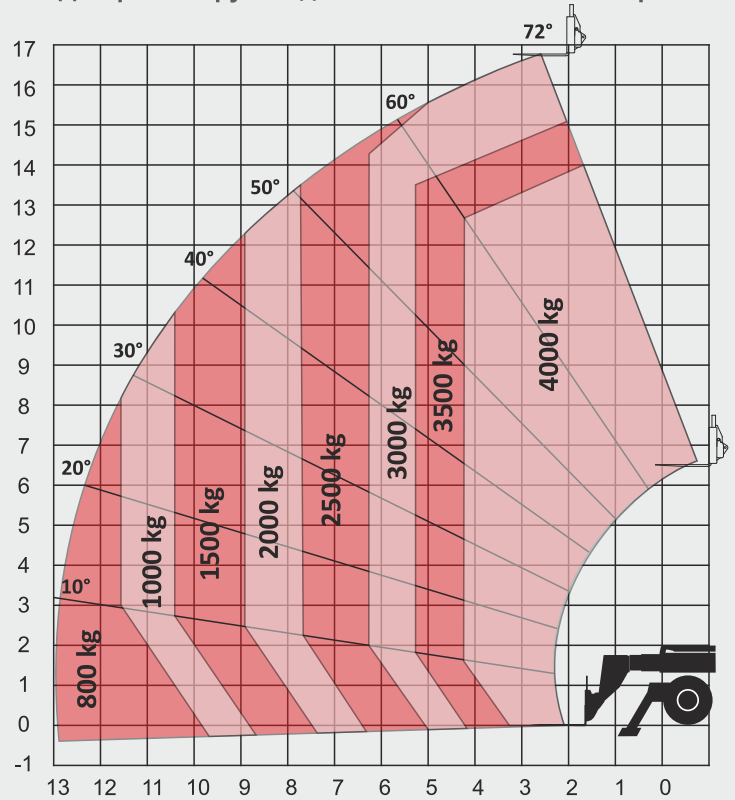
Диаграмма грузоподъемности на стабилизаторах
